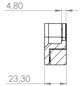
COUPE A-A
