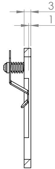
COUPE A-A
